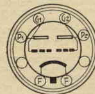
DDD 25 DOPPIO TRIODO B.F. ACCENSIONE 1,2 V. 0,1 A. ANODICA P1-P2: 90 V.
