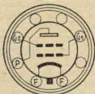
DF 25 PENTODO A.F. ACCENSIONE 1,2 V. 0,025 A. ANODICA 90 V. + GRIGLIA 2 50 V. +
