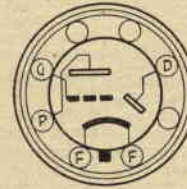
DAC 25 TRIODO-DIODO ACCENSIONE 1,2 V. 0,025 A. PLACCA 90 V.
